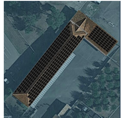
Schéma 3D – implantation centrale
